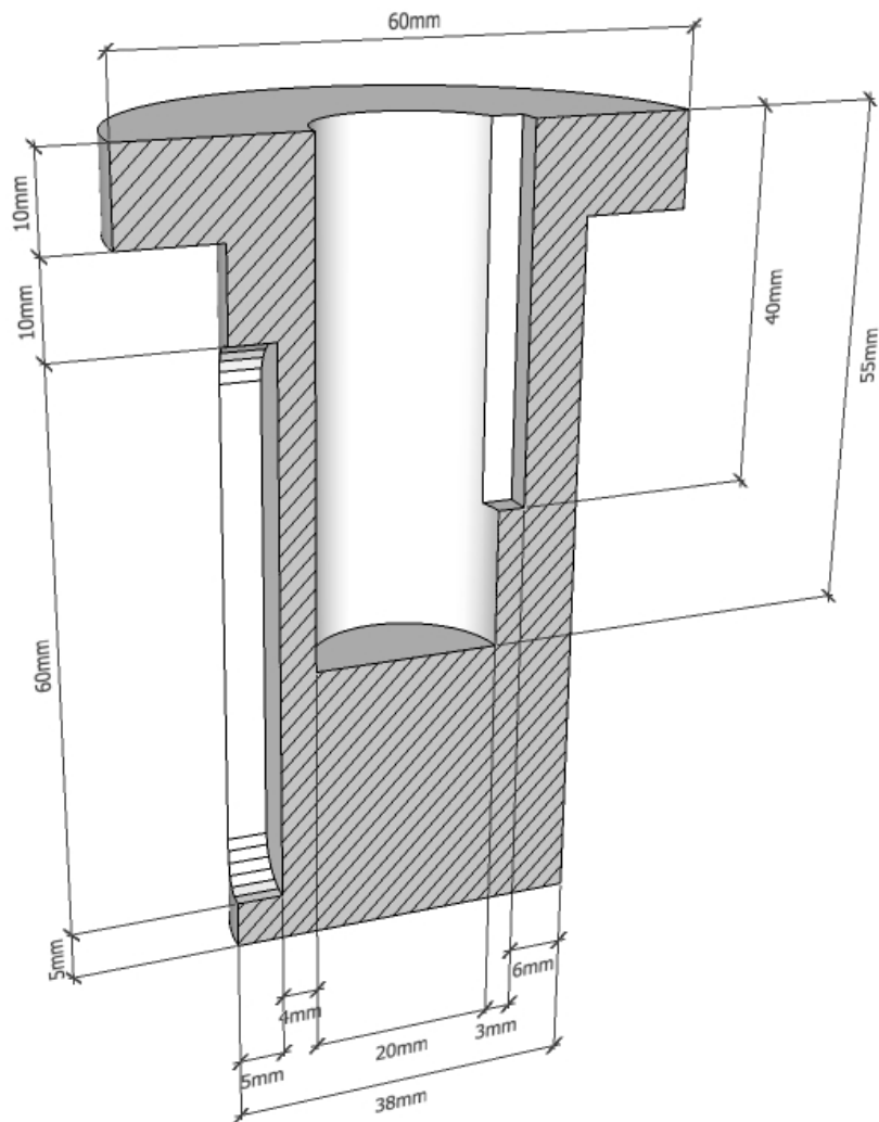
VUE EN COUPE
